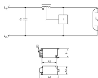
Technische Daten Philips SND 58 220-240V 50/60Hz
